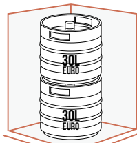
500 mm 610 mm TOT 2 X 30 LITERS EURO GESUPERPONEERD
